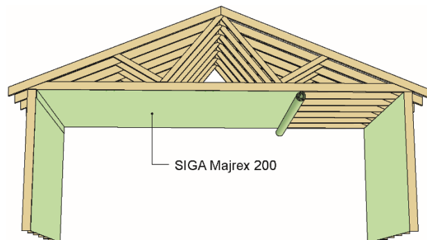
Fig. 1 SIGA Majrex 200 montert i yttervegg og mot kaldt loftsrom
