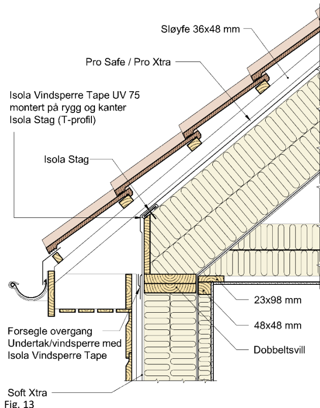
Fig. 13 Eksempel på overgang tak/yttervegg med takutstikk uten gjennomgående sperrer. Overgang undertak/vindsperre forsegles med Isola Tyvek® Vindsperre Tape eller Isola WiFlex Tape med 100 mm bredde.
