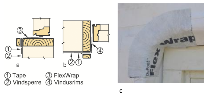
Fig. 6 a-c Tetting rundt inntrukket vindu ved bruk av FlexWrap, Vindsperre Tape og Vindusrim: a) bunnkarm vertikalsnitt b) sidekarm horisontalsnitt c) øvre hjørner forsterket med FlexWrap. Figur 6c: Isola as
