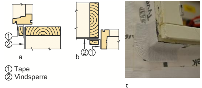
Fig. 8 a-c Tetting rundt vinduer på utsiden av vindsperren ved bruk av Isola Vindsperre Tape: a) bunnkarm vertikalsnitt b) sidekarm horizontalsnitt c) bilde som viser tetting ved karmhjørne ved hjelp av FlexWrap. Figur 8c: Isola as
