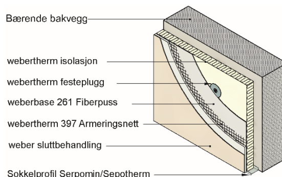
Fig. 1 Oppbygging av weber Serpomin og weber Serpothem fasadesystemer
