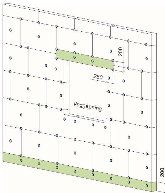
Fig. 2 Brannsikringstiltak i brannklasse 2 for weber Serpotharm over vindu/dør og brannutsatt nedre avslutning
