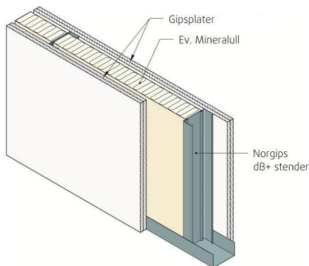
Fig. 1 Prinsipiell oppbygning av Norgips Skilleveggsystem.
