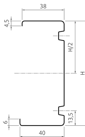
Fig. 2 Norgips C-stender. Profilhøyden H er 68, 70, 75, 95, 100, 120 eller 125 mm
