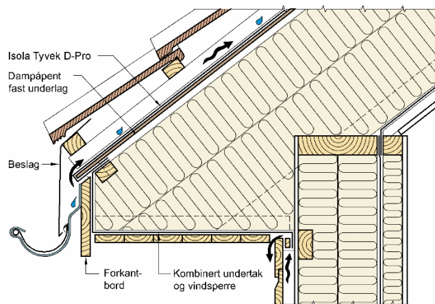
Fig. 5 Eksempel på overgang tak/yttervegg med utstikkende sperrer med Isola Tyvek D-Pro. Isola Tyvek D-Pro føres da rundt hele sperrerfot mot vindsperre på vegg
