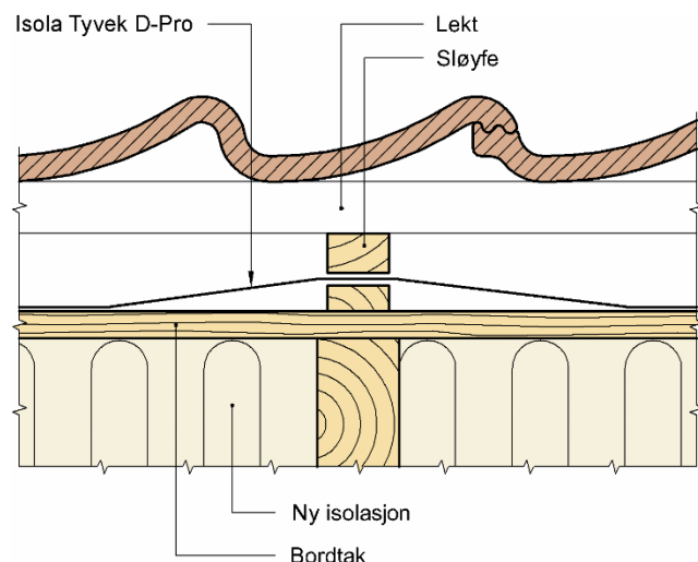
Fig. 9 Isola Tyvek D-Pro lagt på taktro av bord som er isolert på undersiden. Ved ombygning av gamle tak må dampnett papp først fjernes. Lekt under omleggene brukes for å tette omleggsskjøter. Dette er spesielt viktig der hvor underlaget ikke er plant, og hvor skjøtene går på tvers av takbordene. Spesielt for åpne taktekninger som f.eks. skifertak er denne løsningen anbefalt.
