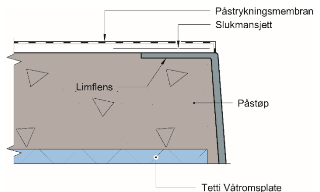
Figur 7 Eksempel på oppbygging av sluk med limflens
