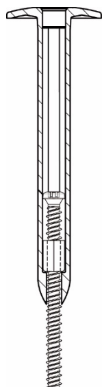
Fig. 26 SFS TIF-N-RH50 Betongskruer med hylse og mutter. Festemidlet er teleskopisk og justerbart.
