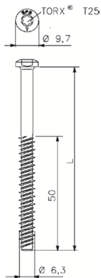
Fig. 25 SFS TI-T25-6-3xL Betongskruer.
