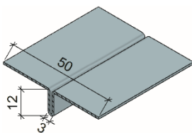
Fig. 7 Profil til Isola Stag. Godstykkelsen er 1,0 mm.
