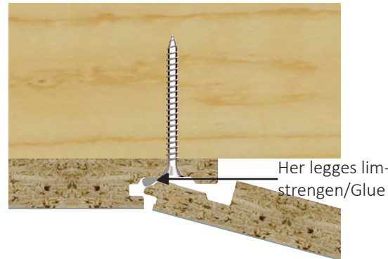
Fig. 2 Låseprofil/Locking profile
